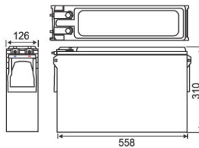
UXP-150F Terminals
