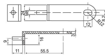
UXP-150F Terminals
