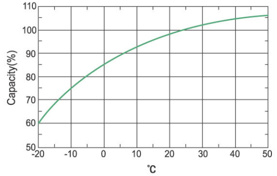
Fig. Ambient Temperature(25°C)
