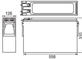
UXP-150F Terminals
