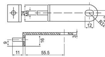
UXP-150F Terminals
